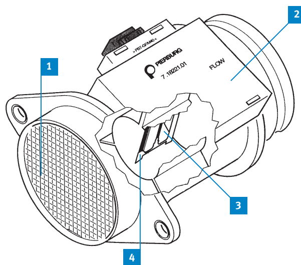
热膜式空气量流传感器 (旧款)
