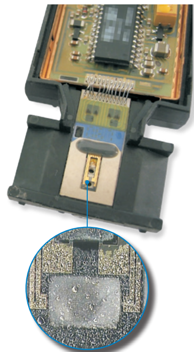
热膜式传感器上存在油雾
